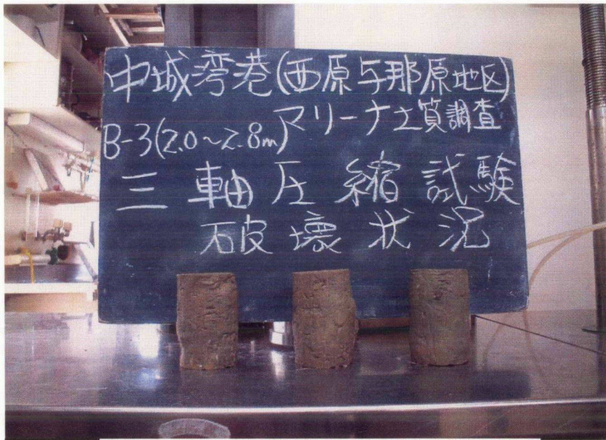
圧縮試験後供試体
