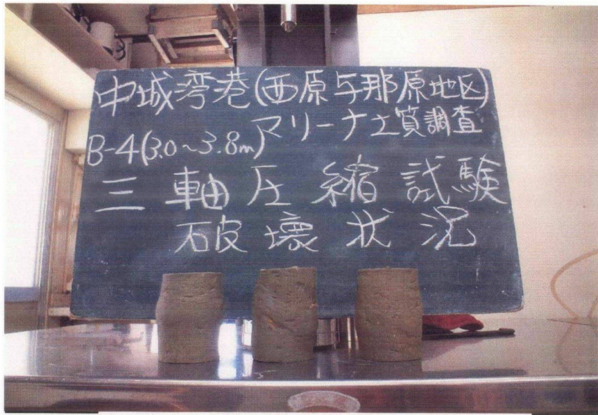
圧縮試験後供試体
