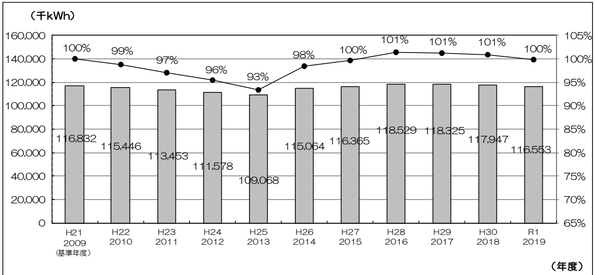
図1.1-1 電気使用量
