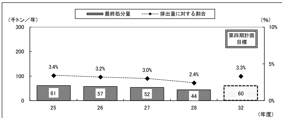
図 2 - 2 2 最終処分量の状況
